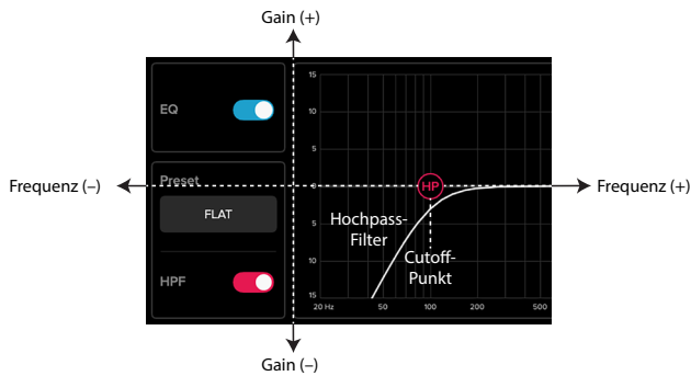
Hochpassfilter aktiviert
